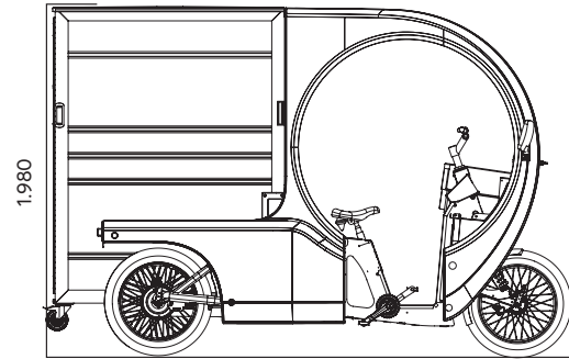
Seitenansicht Box im MovR3
